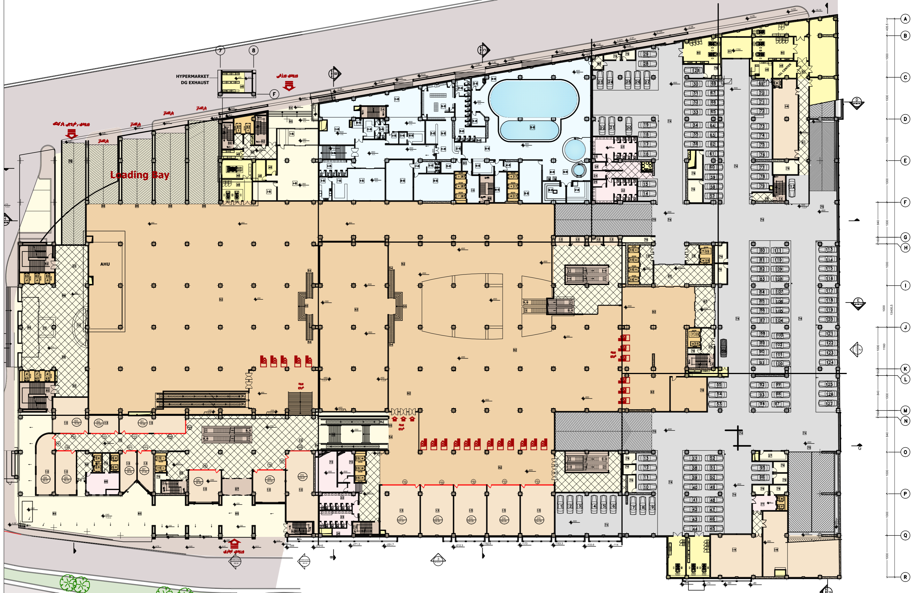
پلان زیرزمین اول
